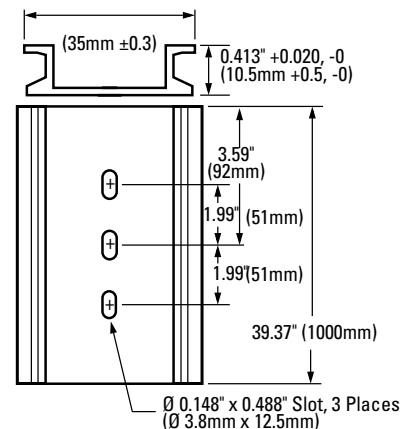
BNDN1000 DIN Rail
