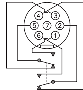
7 PIN MINI CONNECTOR – DCD DPDT FORM CC
