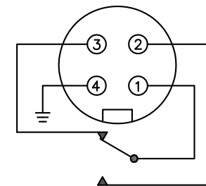
4 PIN MINI CONNECTOR – DCD SPDT FORM C
