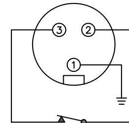
3 PIN MINI CONNECTOR — DCA SPDT FORM B
