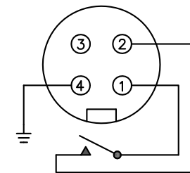
4 PIN MINI CONNECTOR — DCD SPDT FORM A
