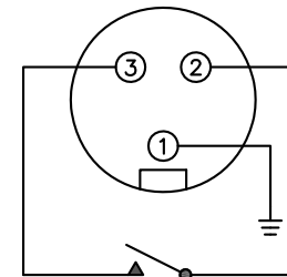
3 PIN MINI CONNECTOR – DCA SPDT FORM A
