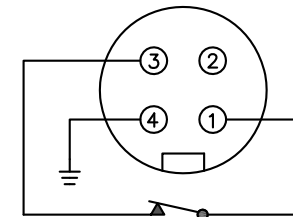
4 PIN MINI CONNECTOR — DCD SPDT FORM B
