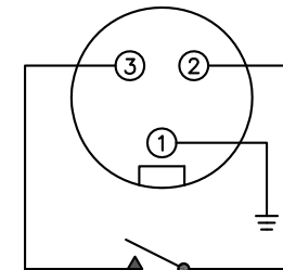
3 PIN MINI CONNECTOR — DCA SPDT FORM A
