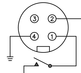
4 PIN MINI CONNECTOR — DCD SPDT FORM A
