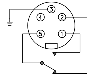
5 PIN MINI CONNECTOR — DCG SPDT FORM C
