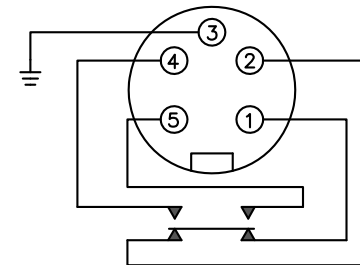
5 PIN MINI CONNECTOR — DCG DMDB FORM Z
