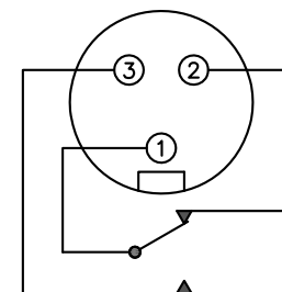
3 PIN MINI CONNECTOR — DCA SPDT FORM C
