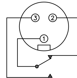
3 PIN MINI CONNECTOR — DCA SPDT FORM C
