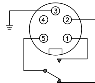
5 PIN MINI CONNECTOR — DCG SPDT FORM C
